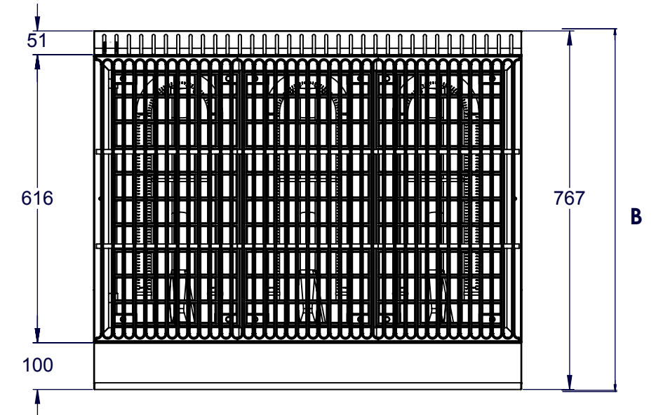
VISTA SUPERIOR
